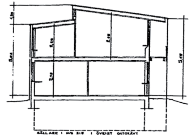
Sektion genom entré
